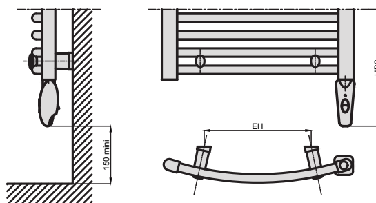
VERSION ELECTRIQUE a liaison RF
